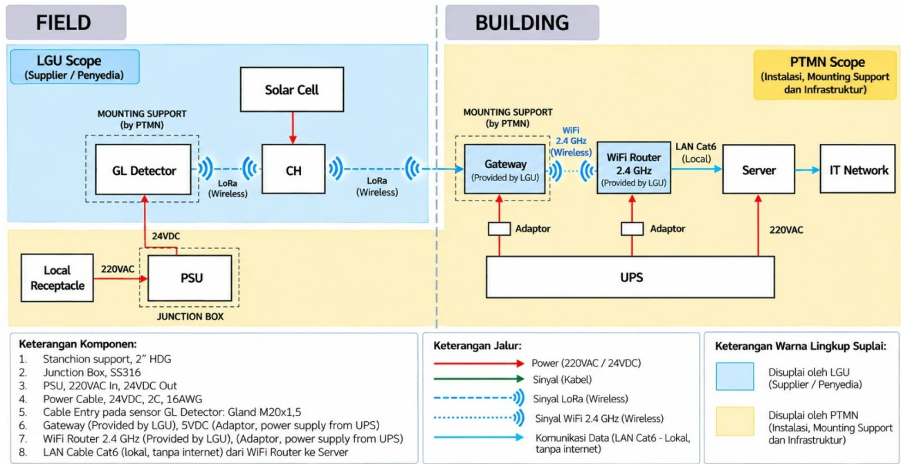
Gambar 2.1 Block diagram lingkup kerja RU IV versi final 8 Oktober 2026 (dari Pertamina RU IV, dilengkapi router Wi-Fi LGU). Biru = disuplai LGU; kuning = disuplai Pertamina (instalasi, mounting support, infrastruktur).
